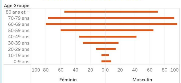
Graphique 3: Distribution des décès par groupe d'âge et sexe du 19 mars 2020 au 29 décembre 2021, Haïti
